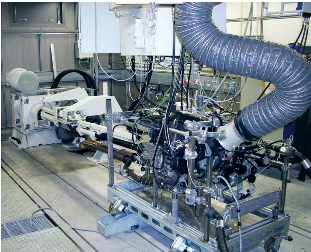
Ein typischer Motoren-Prüfstand
