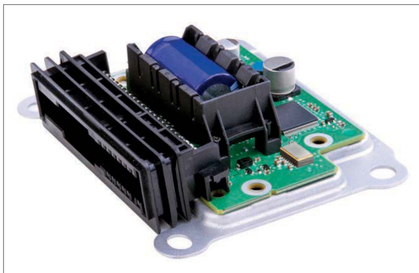
Airbagsteuergerät mit integriertem Sensorcluster
