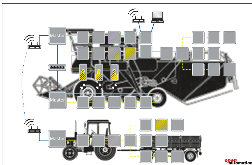
Ethercat als leistungsfähiges Netzwerk mit flexibler Topologie ermöglicht die Vereinfachung der Bordnetzarchitektur. Fahrzeuge können miteinander, zum Beispiel über Funk, gekoppelt werden.
