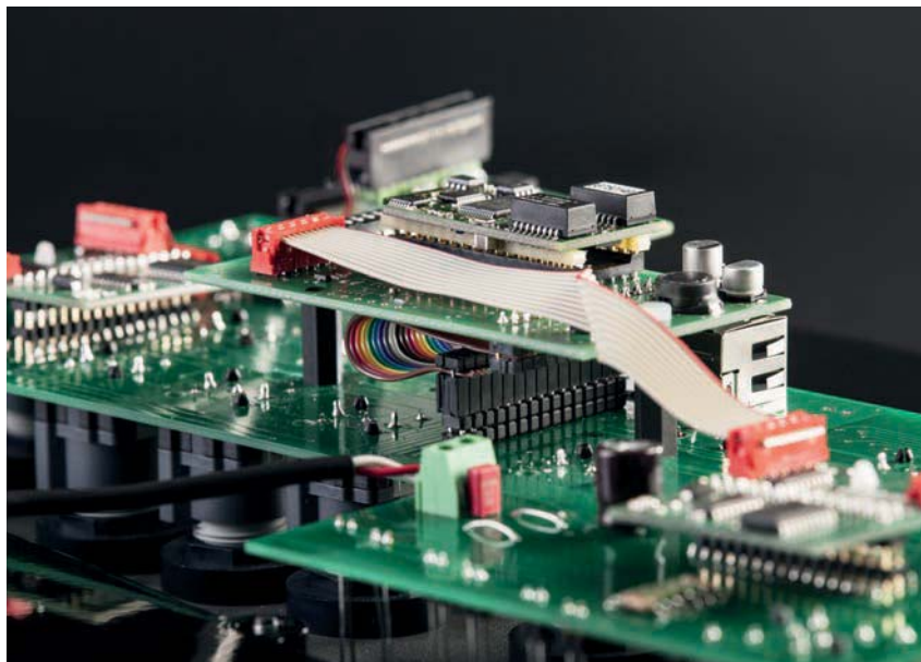
Blick auf die Rückseite des Bedienpanels: Auf der Trägerkarte sitzt die Adapterplatine mit dem standardisierten Stecksocket für die Unigate-IC-Busmodule.
