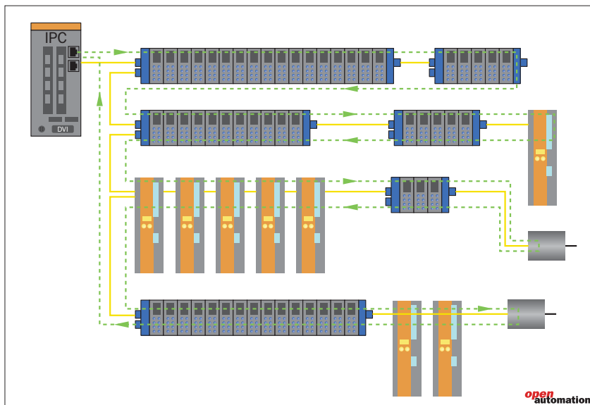
Die logische Weiterleitung der Ethernet-Frames erfolgt mittels des ESC (Ethercat Slave Controller).
