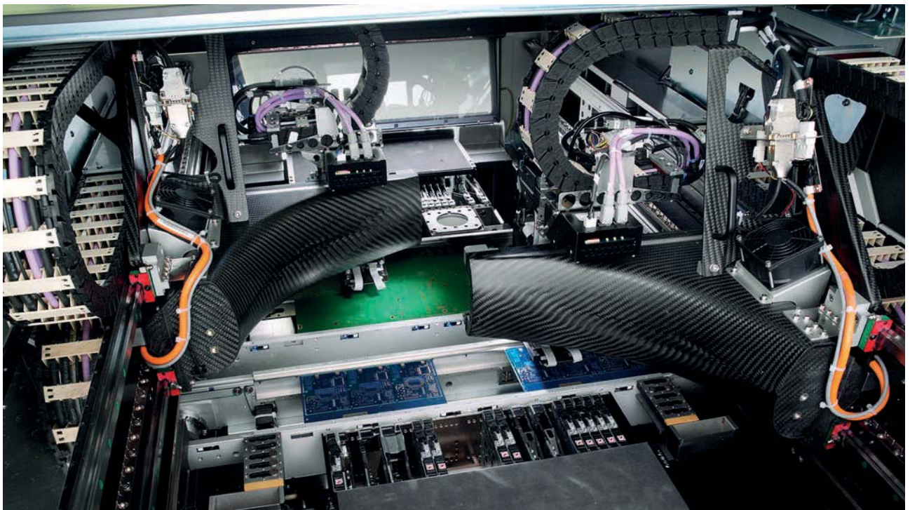
Bestens geeignet für die Bestückung auch bei hohem Produktmix: die iFlex T2 von Assembléon
