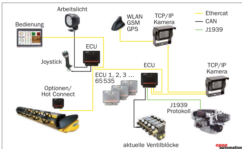
Schrittweise Migration durch Einbindung von vorhandenen Netzwerken in das Ethercat-Netz
